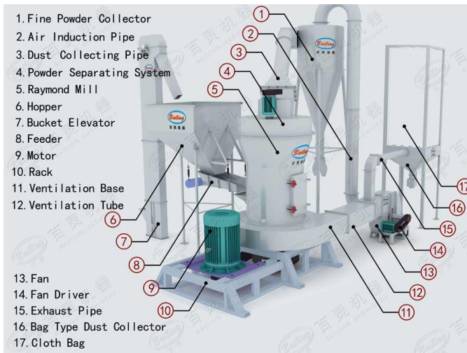
Figura 8. Ilustración de la instalación completa del molino tipo Raymond (Recuperado de : http://www.ascendme.com/mill/82.html ).
